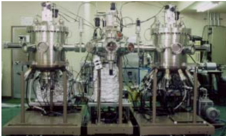
マルチチャンバMBE装置
