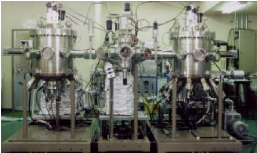
Si and InGaPN 用 MBE 装置 (RC2100M)
